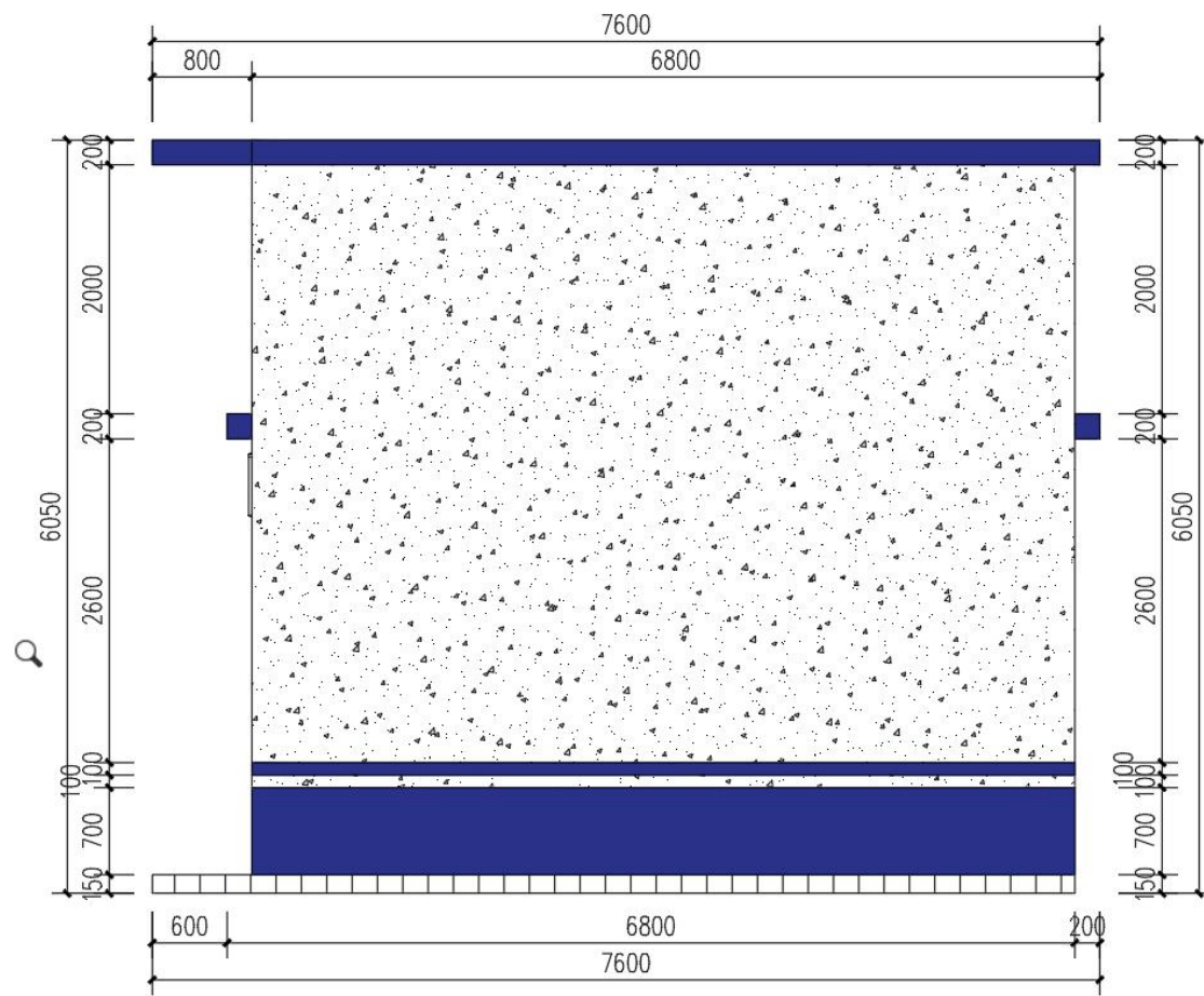
食堂右立面图
