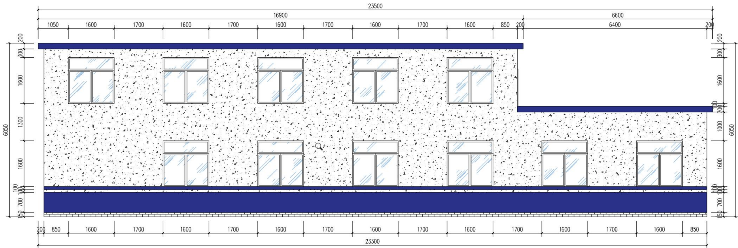
食堂后立面图
