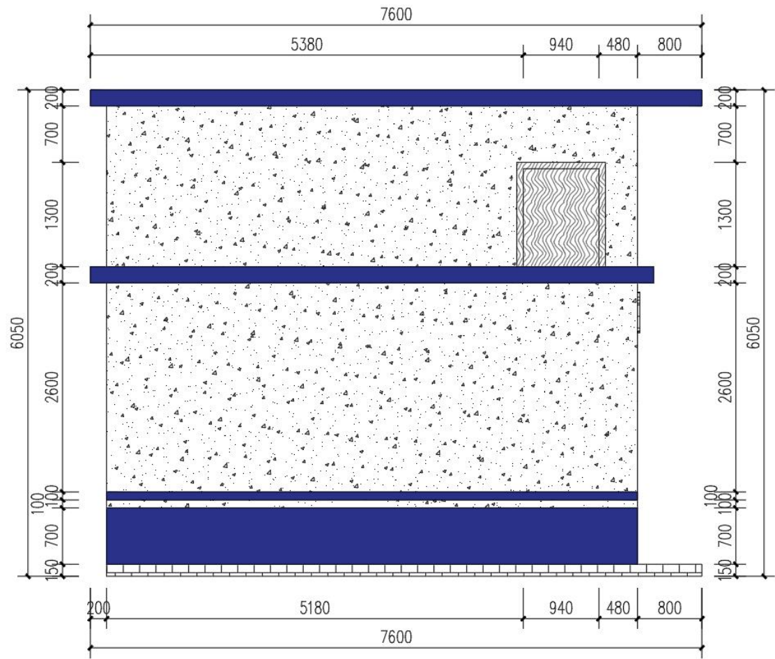
食堂左立面图
