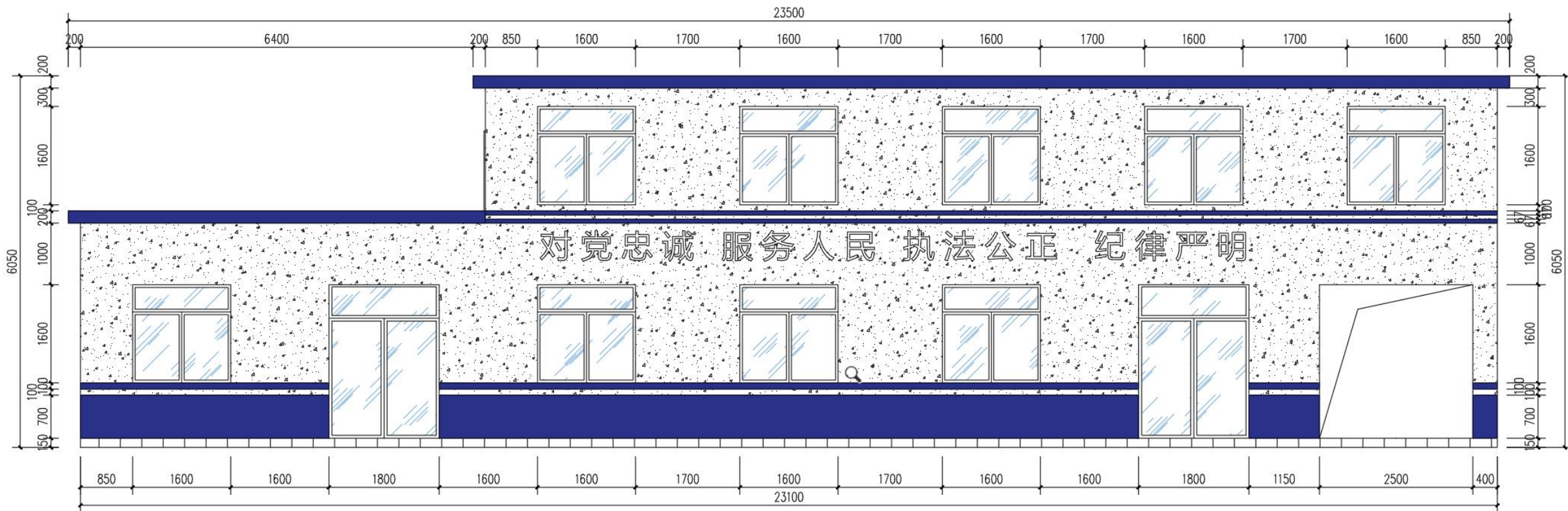
食堂正立面图
