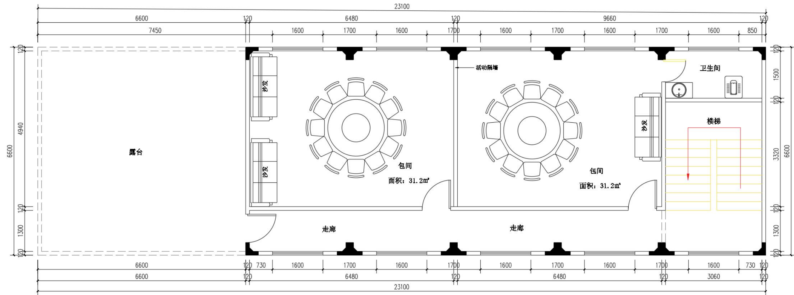
食堂二楼平面图
